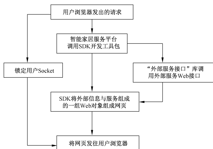
图 A.2 外部设备调用服务界面流程图
