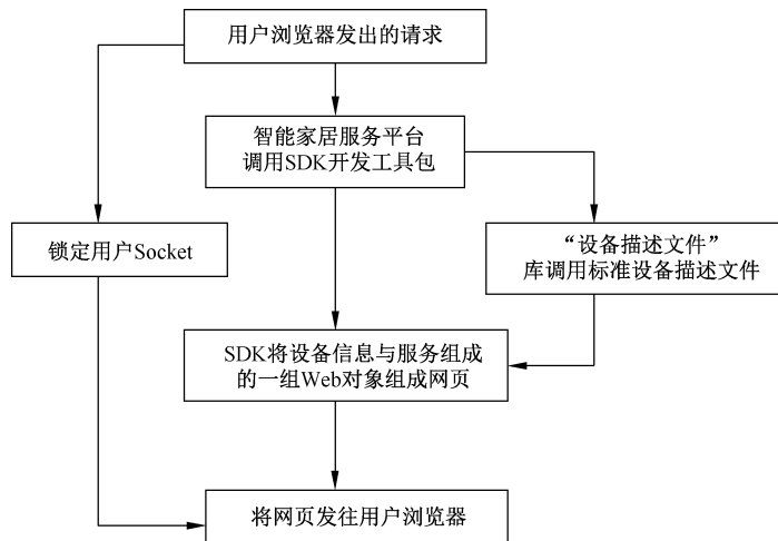
图 A.1 内部设备调用服务界面流程图
